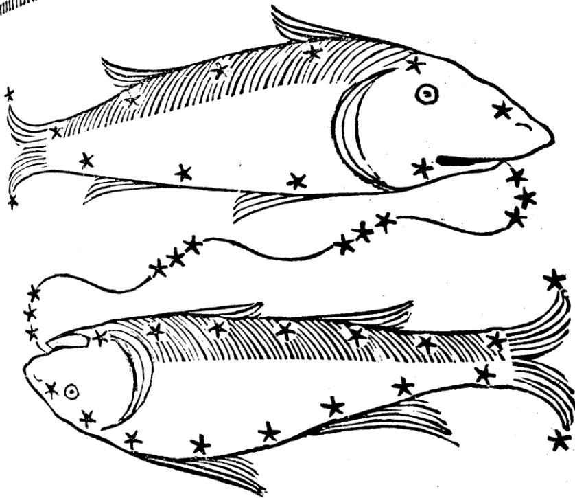
Pisces
