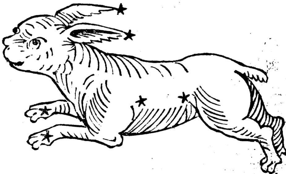
Lepus
